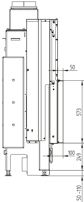
Telaio 78/57 4 lati 80 mm
